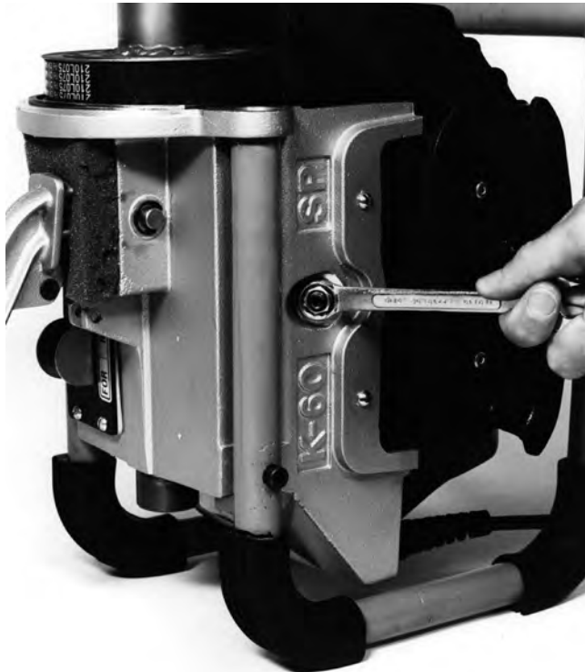
Figura 13 – Afloje la tuerca de inmovilización
